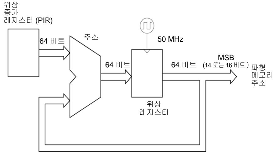
위상 어큐뮬레이터 회로도
