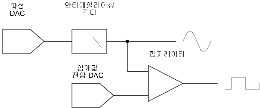
방형파 생성 회로도
