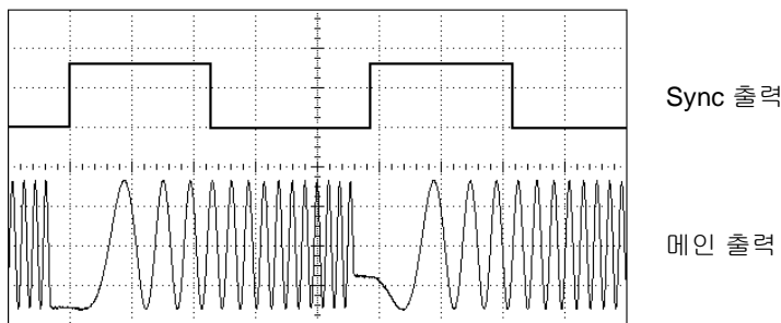
주파수 스위프
