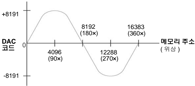
파형 메모리의 사인과 형태
