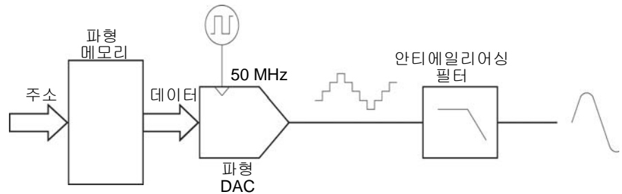
직접 디지털 합성 회로도
