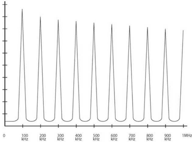
위 파형의 스펙트럼 (100 kHz)
